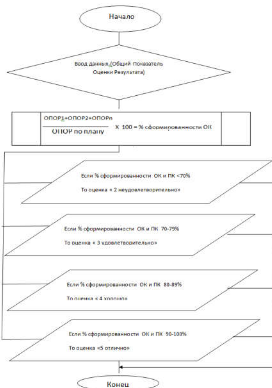
Рис. 8. Алгоритм расчета итоговой оценки ДП
